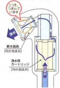
本体の断面図
